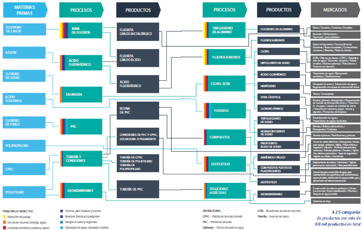
Diagrama de procesos, productos y usos (1.2, 2.3)
